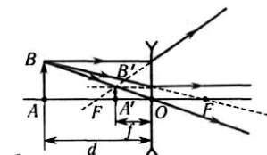
рассеивающая линза
